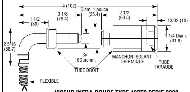
WISEUR INFRA-ROUGE TYPE 48PT2 SERIE 9000
