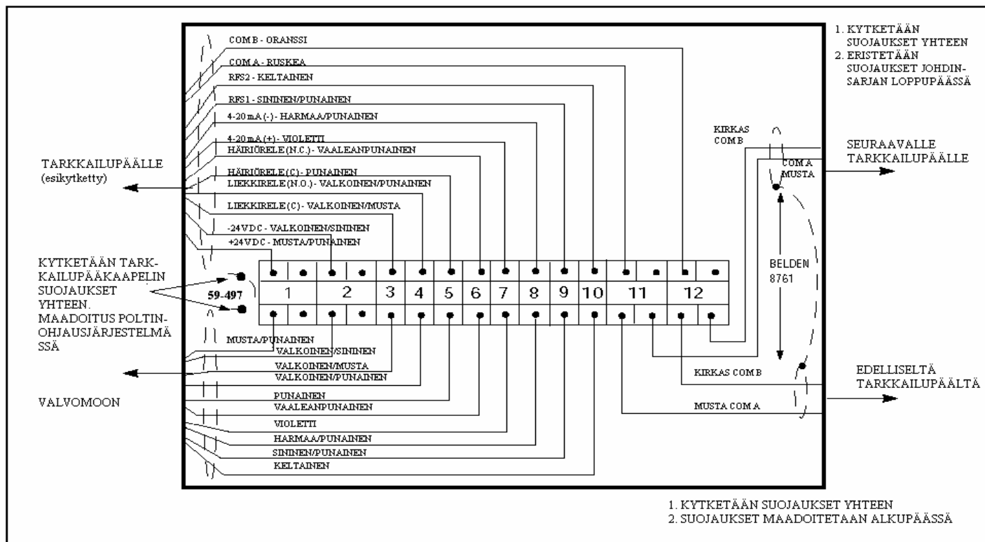
KUVA 21. JOHDOTUSKAAVIO JOHDINSARJALLE
