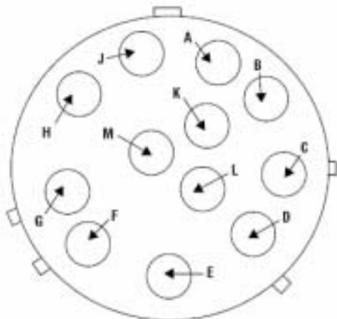
KUVA 17. PIKALIITINPISTIKKEET
