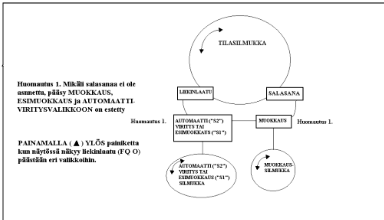
KUVA 23. TARKKAILUPÄÄN VALIKKORAKENNE
