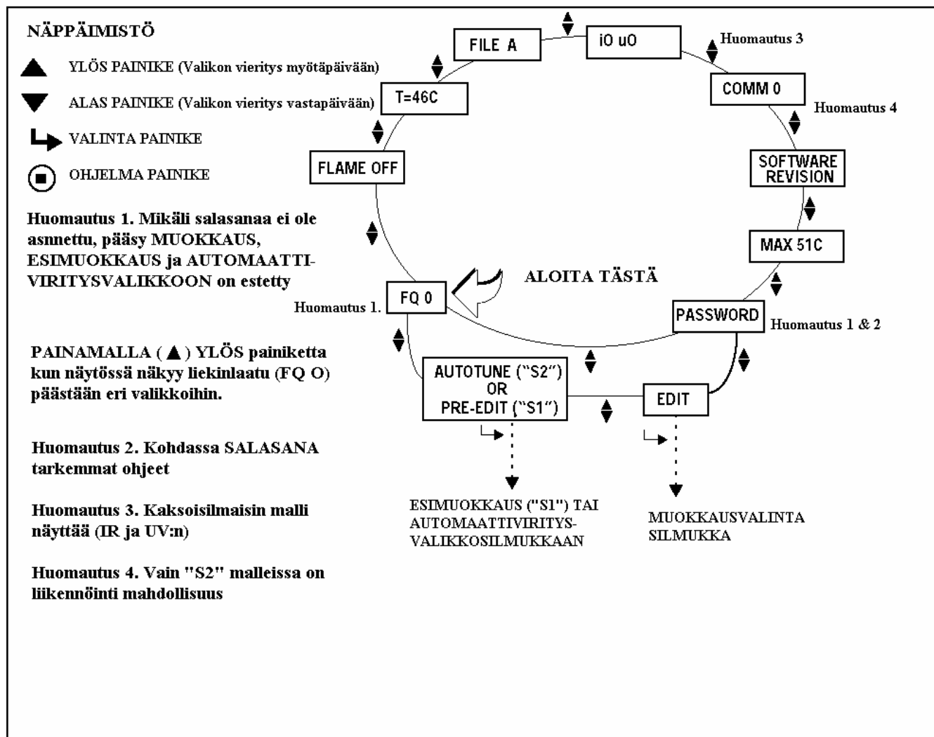
KUVA 25. TILAVALIKKO
