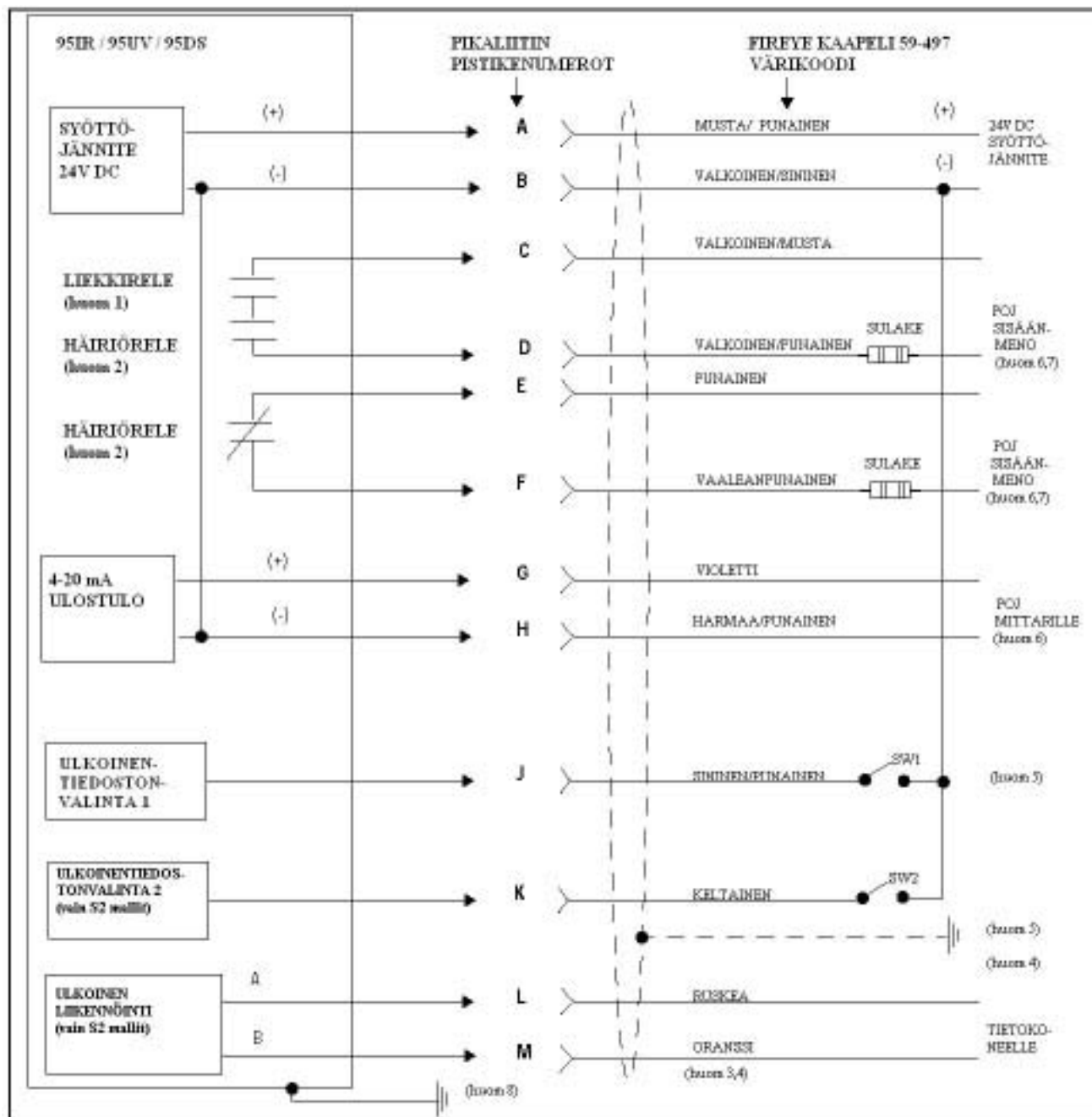
KUVA 13. TARKKAILUPÄÄN KYTKENTÄKAAVIO
