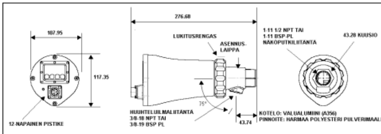
KUVA 2. 95IR/95UV/95DS TARKKAILUPÄÄT "CG" MALLIT 3 m:n KAAPELILLA
