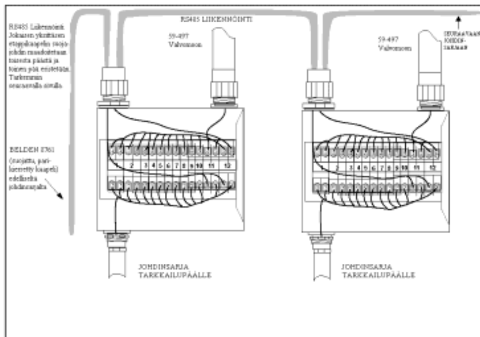
KUVA 21. JOHDOTUSKAAVIO JOHDINSARJALLE
