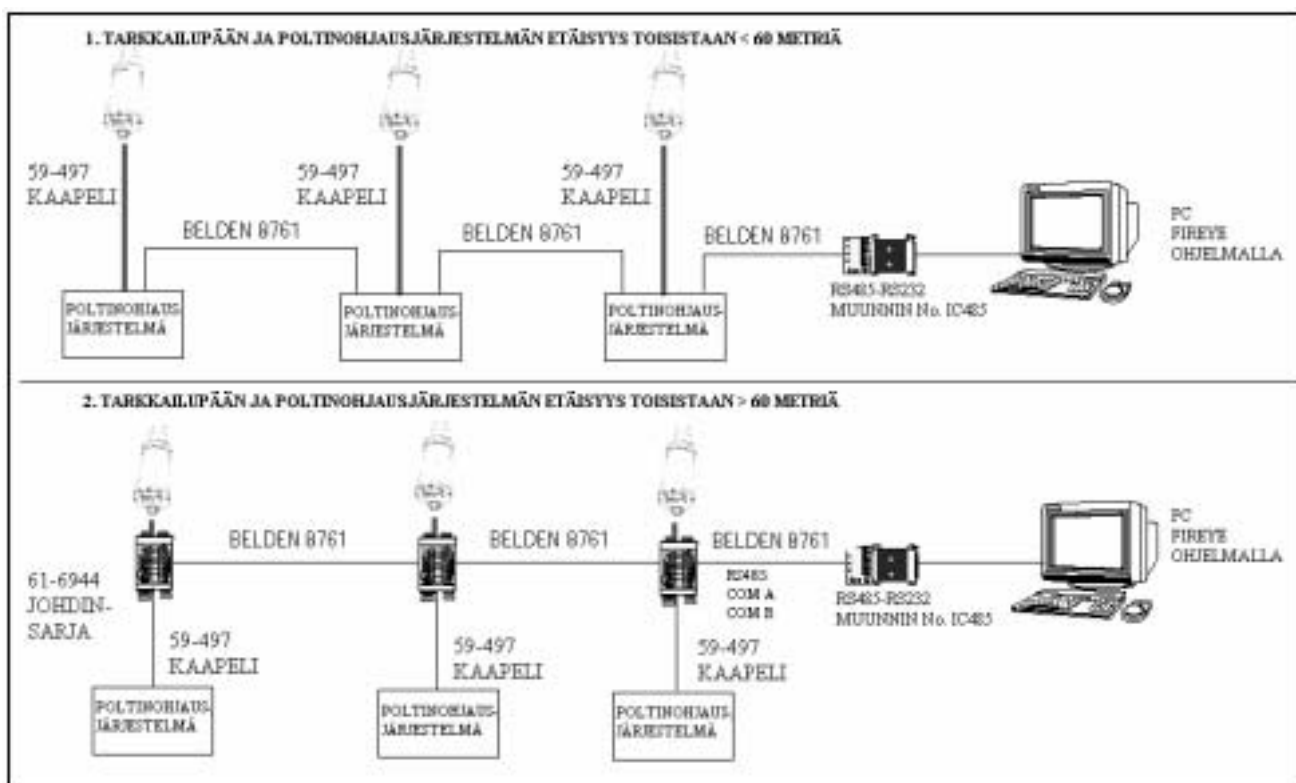
KUVA 19. KAUKOLIIKENNEKAPELOINTI
